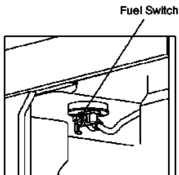
Топливный кран
