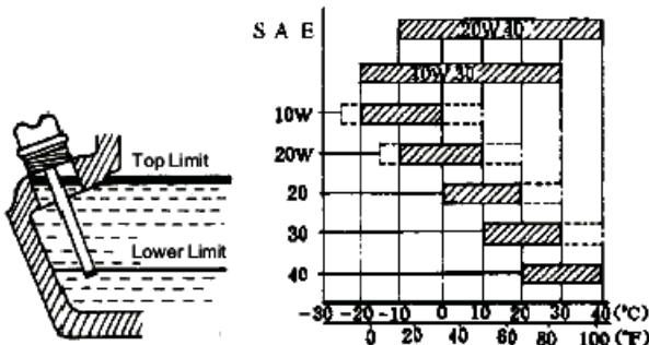
Уровень масла
